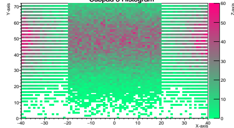
Subpad 6 Histogram
