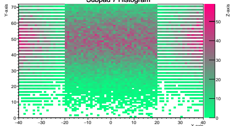
Subpad 7 Histogram
