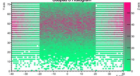
Subpad 8 Histogram
