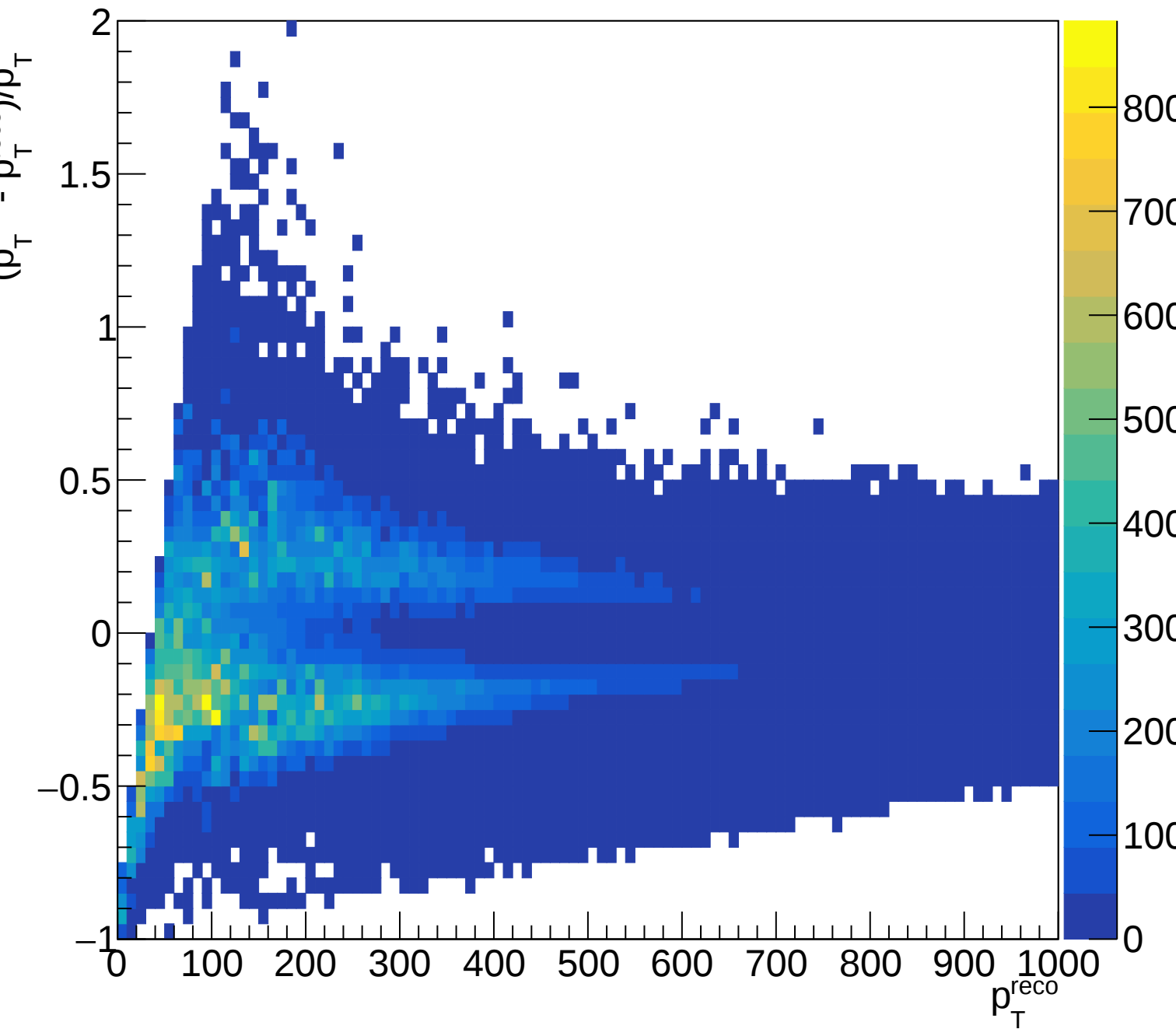
AnyJetPtDeviation_central_reb_vs_reco
