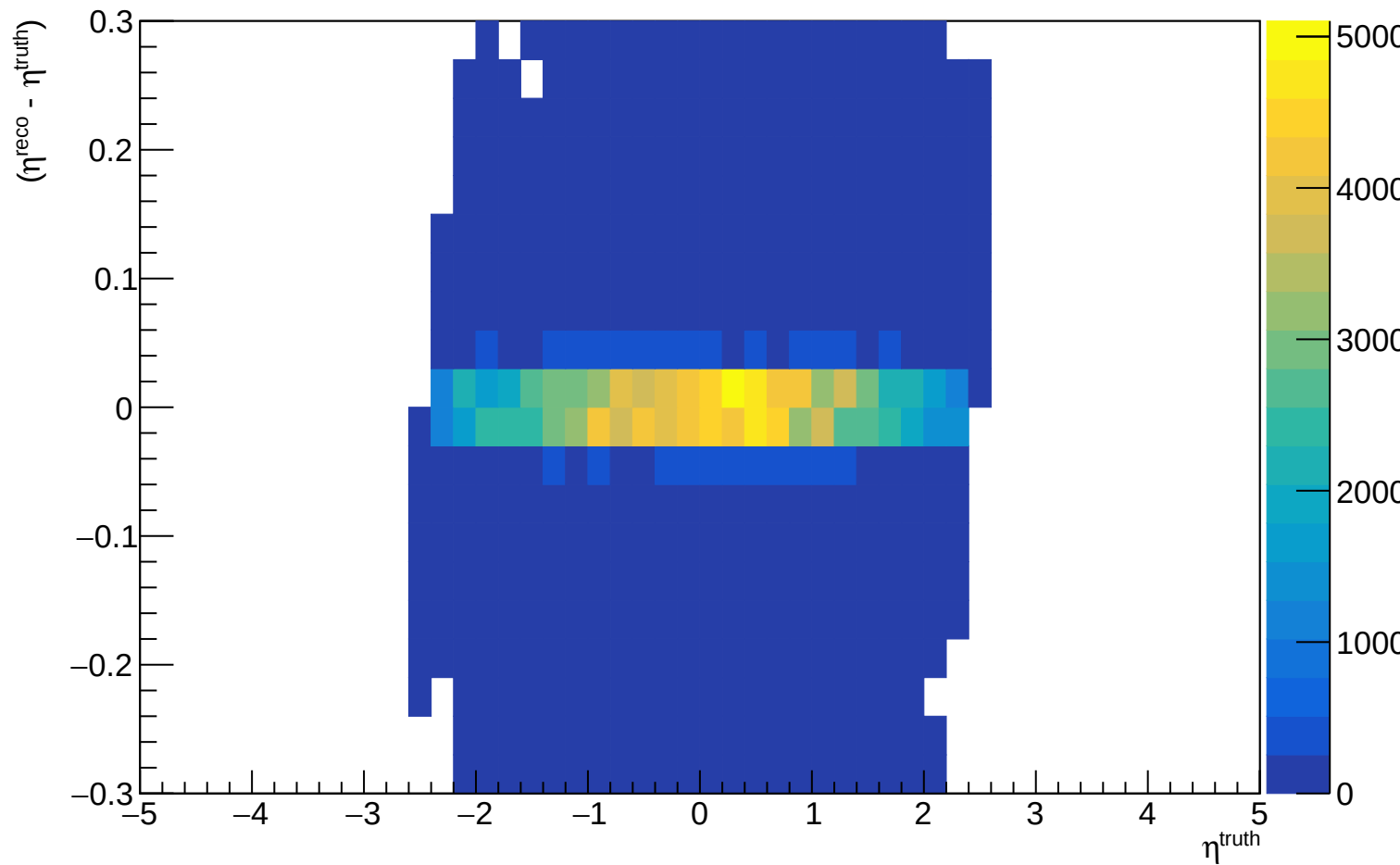
AnyJetEtaDeviation_central_reco_vs_truth
