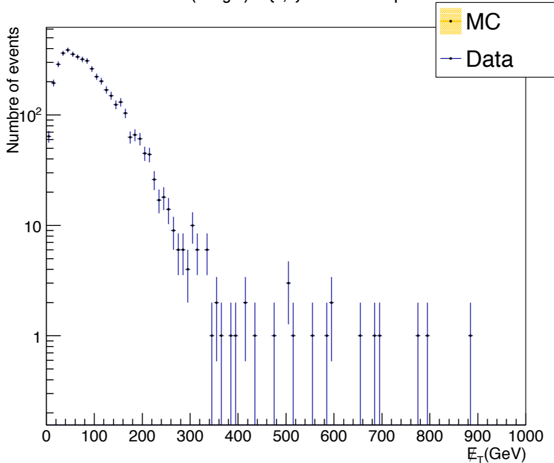
MET Data/MC(Weight) ID{1,5} letal< 2.4 mupt > 50 Gev
