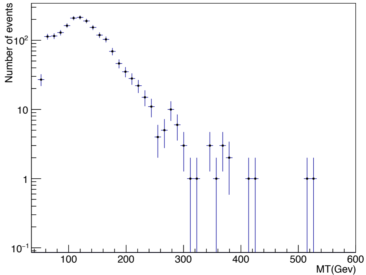
MET Data/MC(Weight) ID{1,5} letal< 2.4 mupt > 50 Gev
