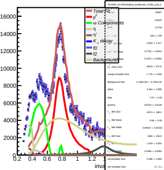
p T bin 2.2 - 2.6 GeV/c
