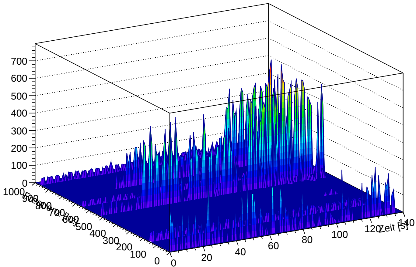
Vibrationsspektrum Weiterlauf CH1, Farben: Amplitude [arb. units]
